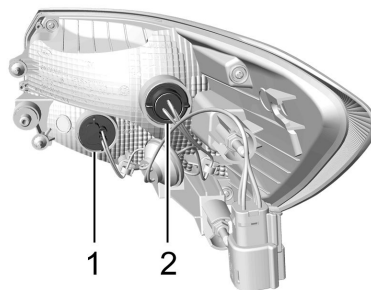
Se muestra el lado del conductor (versión sin LED). El lado del acompañante es similar
