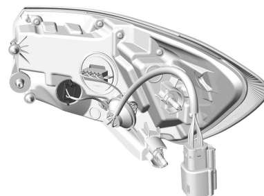
Se muestra el lado del conductor (versión con LED). El lado del acompañante es similar
